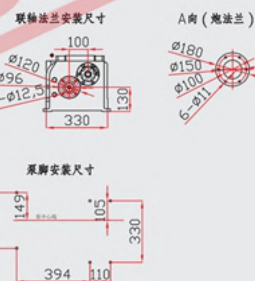
安装尺寸 / Installation dimension
