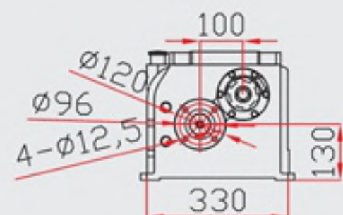
联轴法兰安装尺寸
