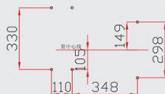
泵脚安装尺寸
