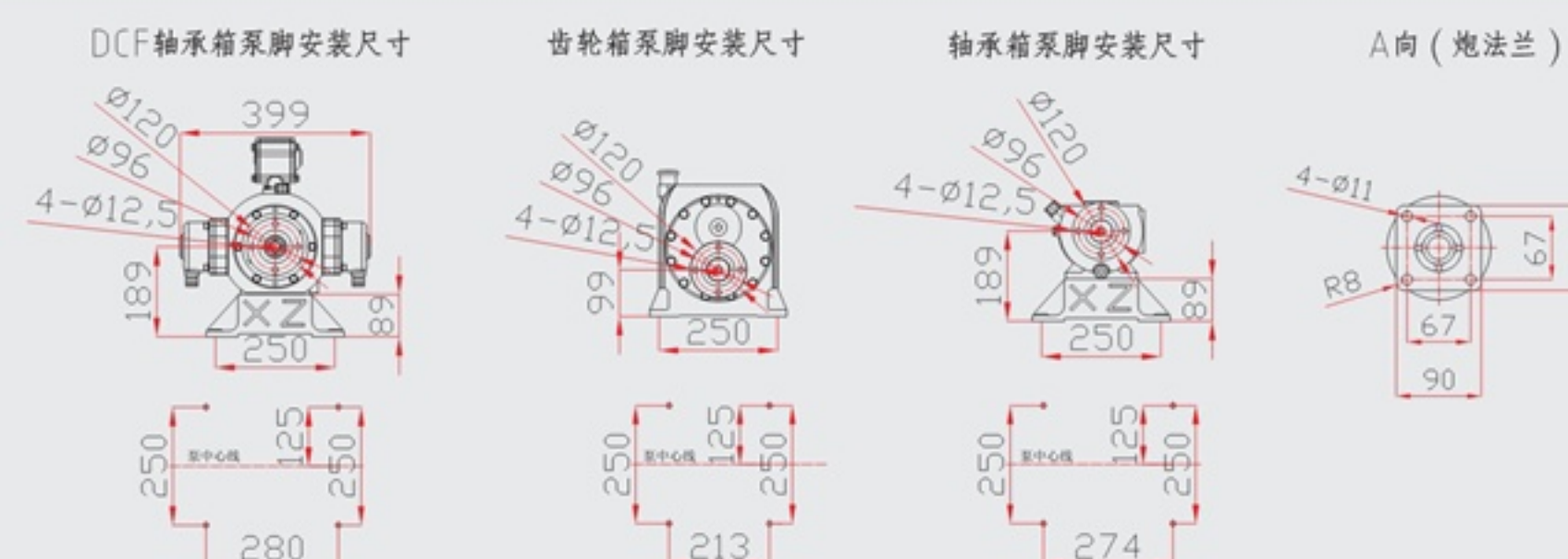
安装尺寸 / Installation dimension
